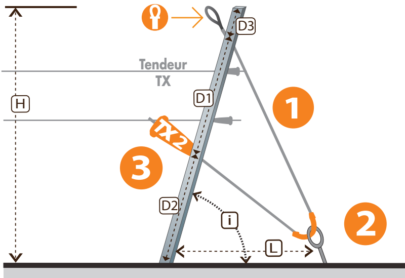
Schéma d'installation du Kit Amarre sur piquet Métal
